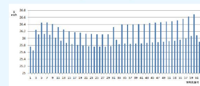
各导风孔风量 Air volume of each air outlet
