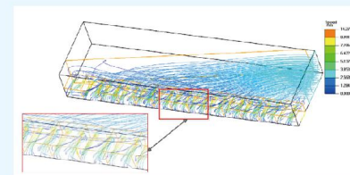
速度流线 Air speed motion pattern
