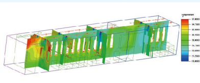
温度云图 Temperature
