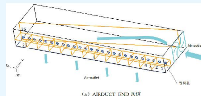
风道模型 Air duct model
