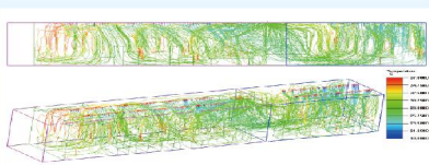
速度流线 Air speed motion pattern
